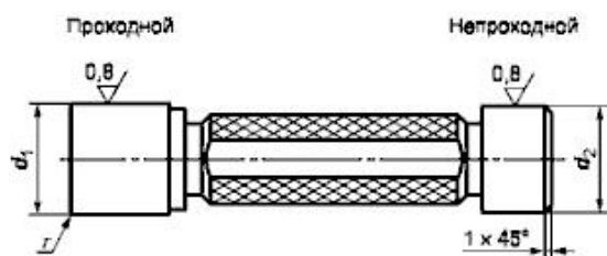
Рисунок А.2 - Проходные и непроходные калибры-пробки для контроля охватывающих концов фитингов
